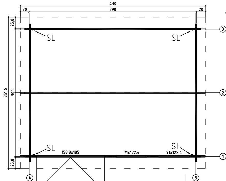
GROUNDPLAN - GRUNDPLAN - PLAN DE MASSE
