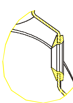
Coupe du joint DN 50 monté
